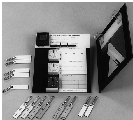
Abb. 3.3.1/2h): Fa. Magin, einzelne Überwachungstafel
