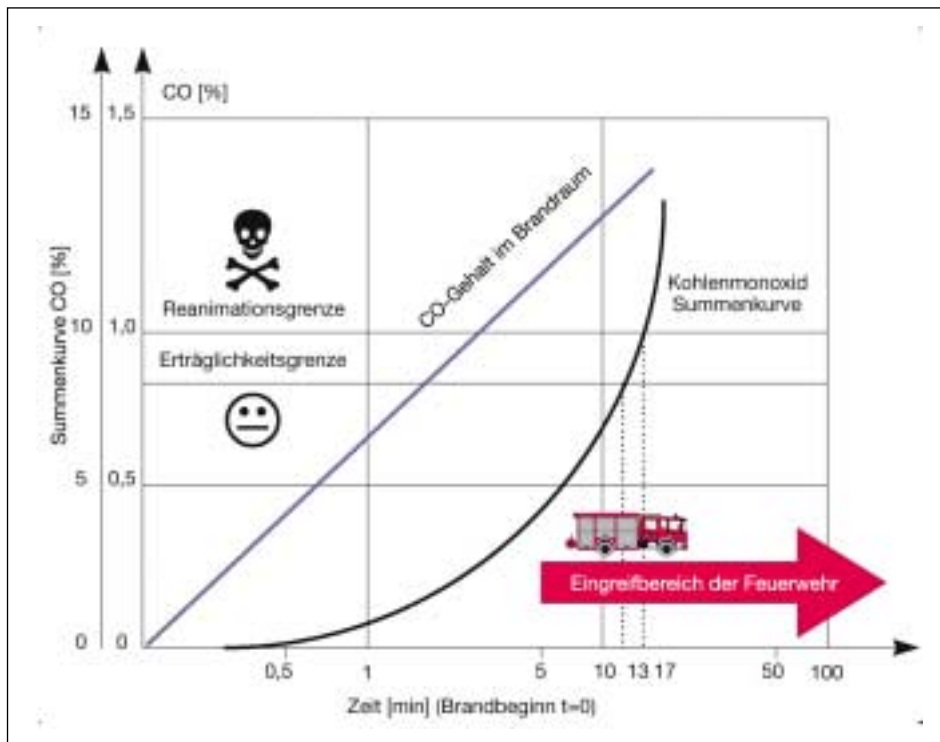
Abb. 11.1.3/1: Überlebenszeiten im Brandrauch (Grafik: de Vries)
