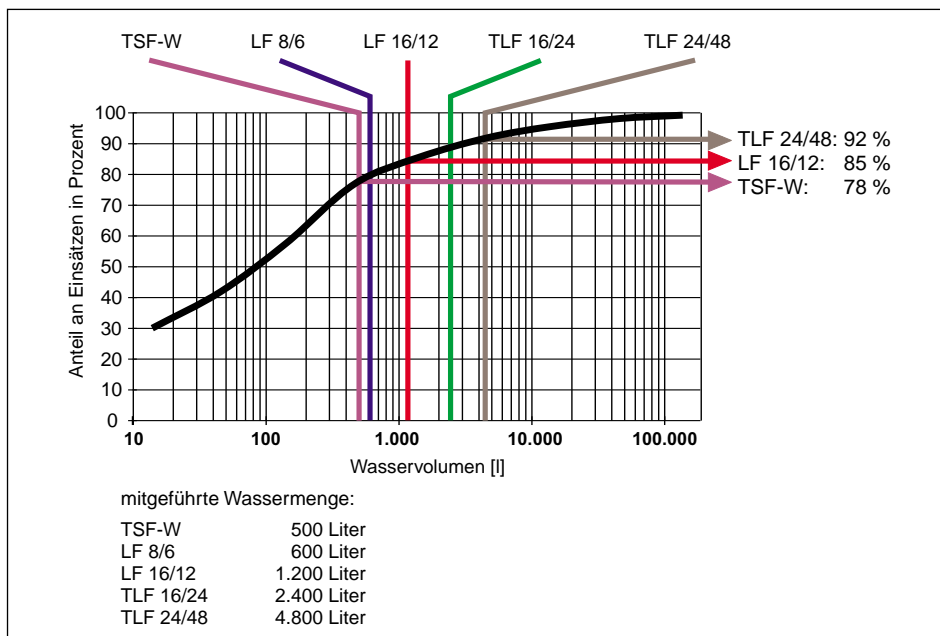
Abb. 13.1.1/2: Verbrauchshäufigkeit verschiedener Wassermengen und Löschwasservorrat von in Deutschland genormten Löschfahrzeugen (Grafik: de Vries)
