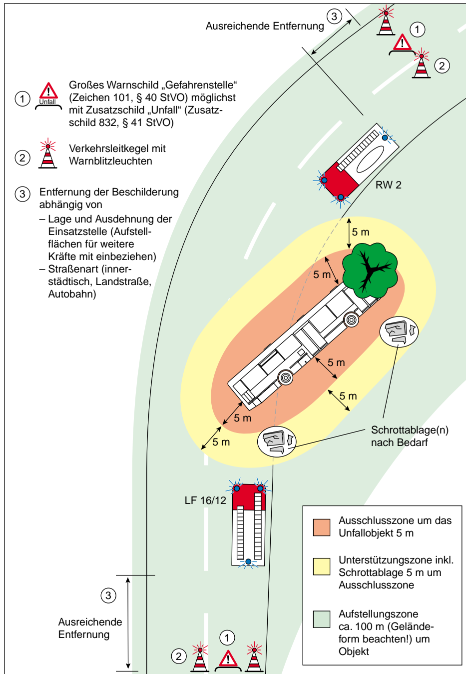
Abb. 2.3/4: Absperurmaßnahmen und Absperrbereiche bei einem Busunfall (Grafik: Cimolino, vgl. CIMOLINO, U., 2000)
