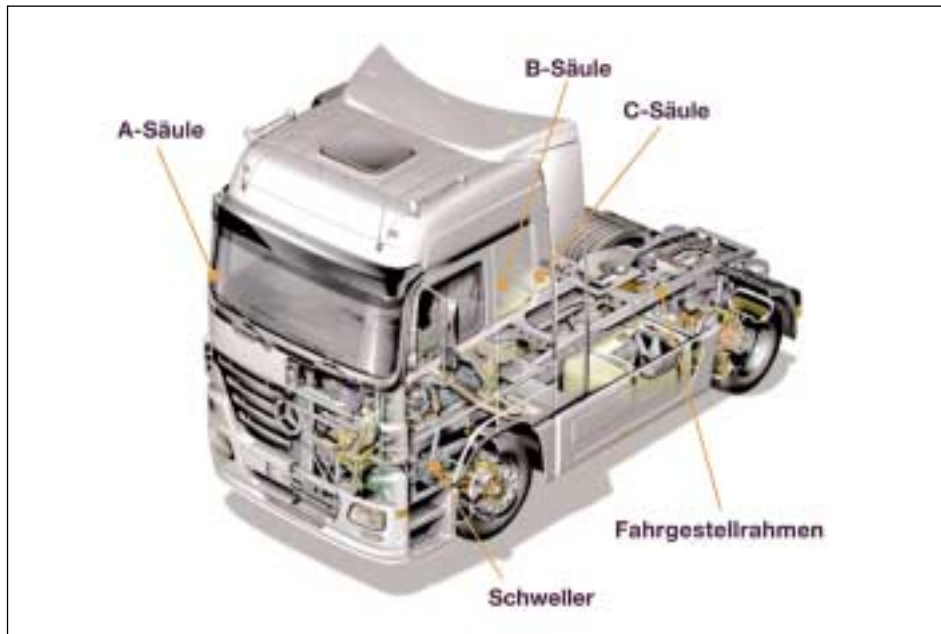
Abb. 3.3.1/1: Mercedes-Benz Actros Sattelzugmaschine (inkl. Fahrerhaus) mit eingezeichneten Benennungen (Grafik: DaimlerChrysler)
