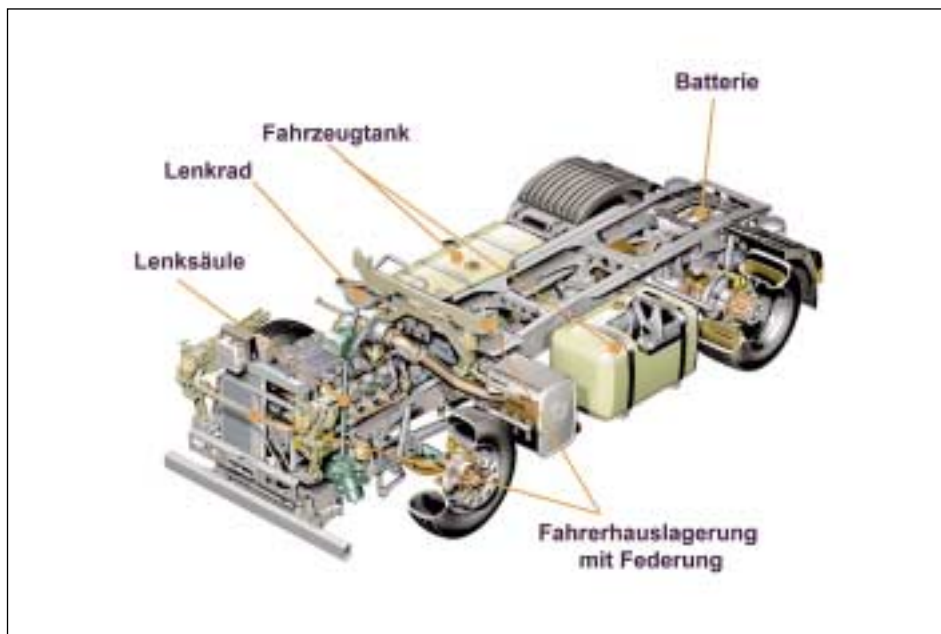
Abb. 3.3.1/2: Mercedes-Benz Actros Sattelzugmaschine (ohne Fahrerhaus) mit eingezeichneten Benennungen (Grafik: DaimlerChrysler)
