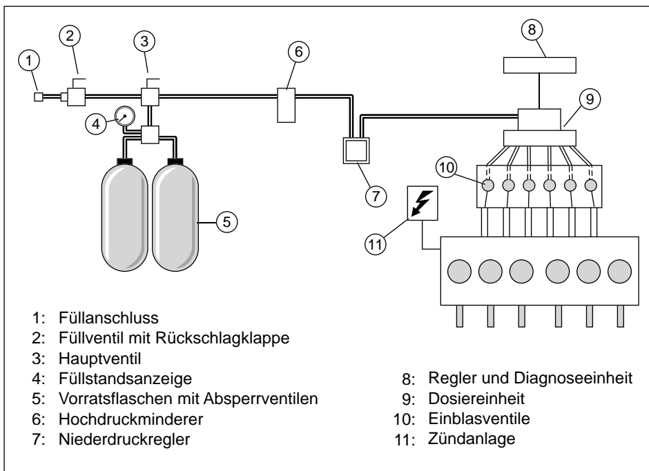
Abb. 3.5.3/6: Schematische Darstellung einer Erdgasanlage (Grafik: Cimolino, vgl. KOLB, T., 1995)
