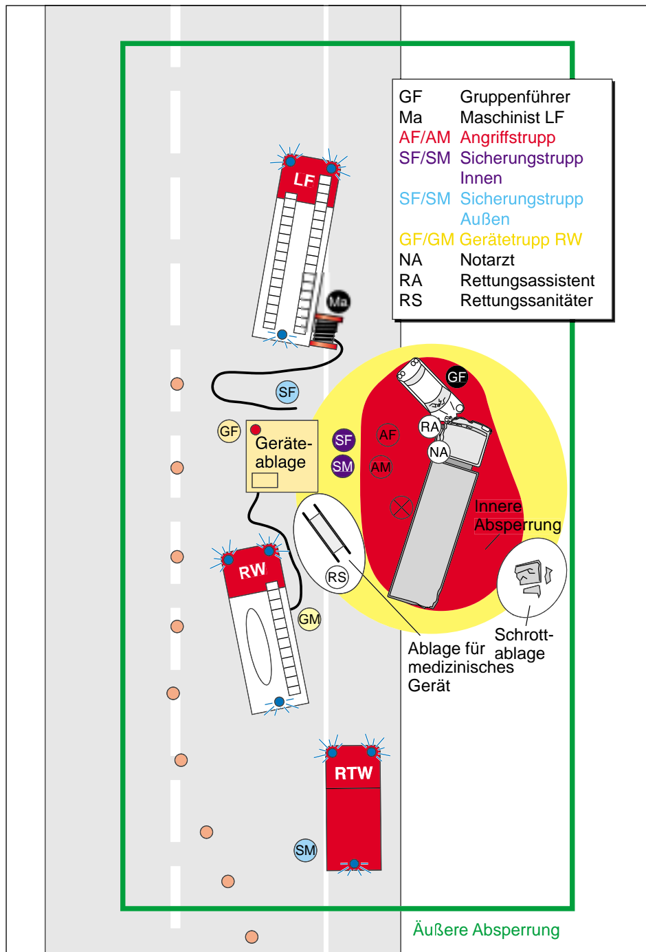
Abb. 6.5.1/1: Personal- und Einsatzstellengliederung (Grafik: Südmerse)
