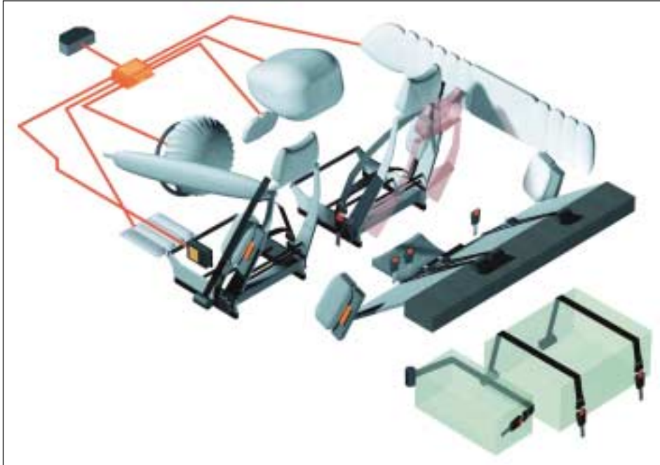
Abb 3.2.1.3/1: Mögliche Airbagvarianten (Grafik: Autoliv)
