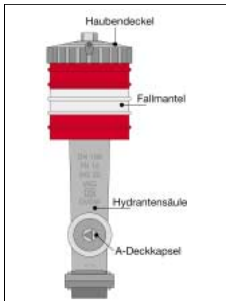
Abb. 3.3.2/24: Überflurhydrant geschlossen (Grafik: Freynik)
