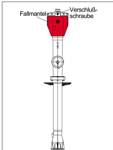
Abb. 3.3.2/26: Überflurhydrant moderner Gestaltung (Teilschnitt) (Grafik: VAW-Armaturen GmbH)
