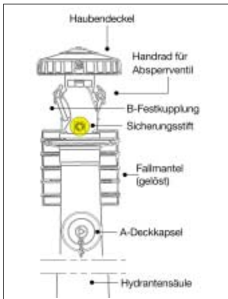
Abb. 3.3.2/23: Überflurhydrant mit gelöstem Fallmantel (Grafik: Freynik)
